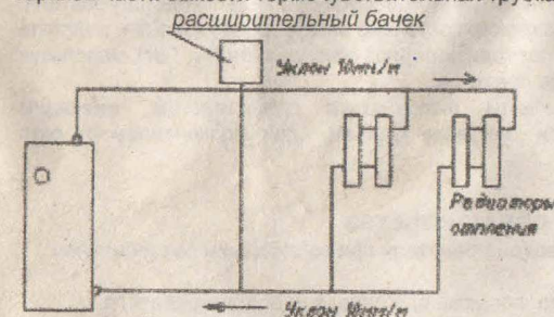
Рис.1. Схема монтажа открытой системы отопления
