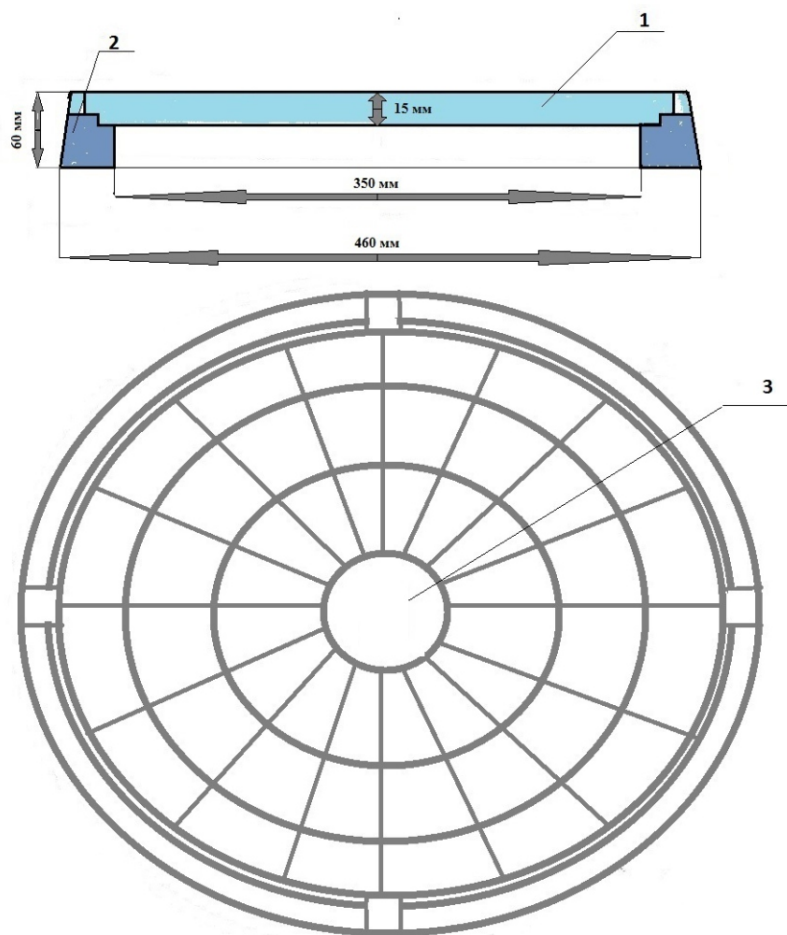
1-крышка, 2-корпус, 3-обозначение типа люка.
