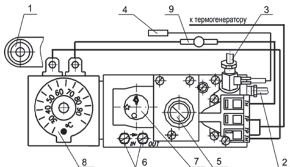
Рис. 9. Блок управления
