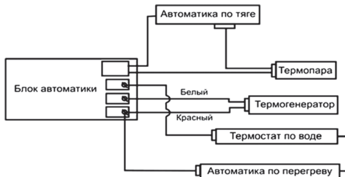
Рис. 11. Схема электроподсоединений блока автоматики от 40 до 70 кВт
