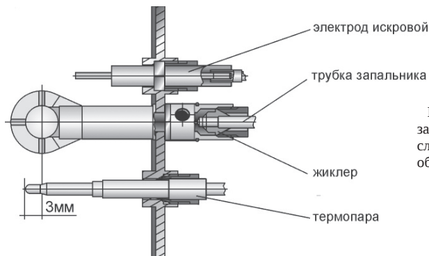
Рис. 3. Запальная горелка
