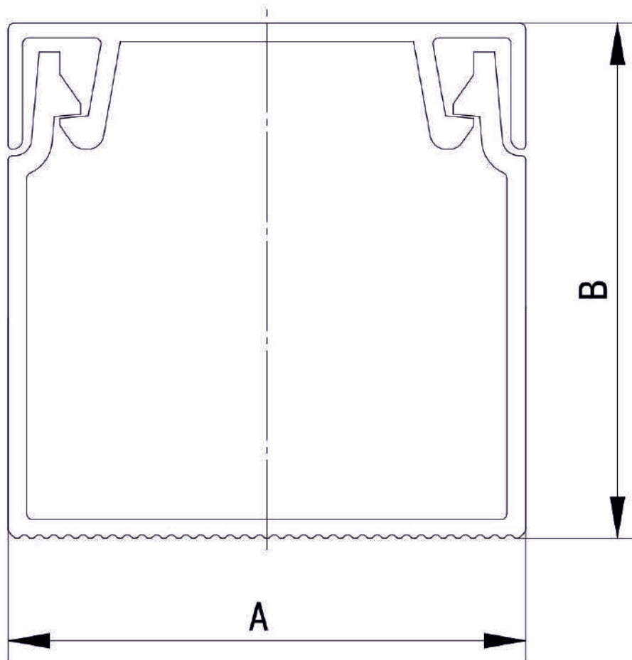
Рисунок 1. Габаритные размеры кабель-канала
