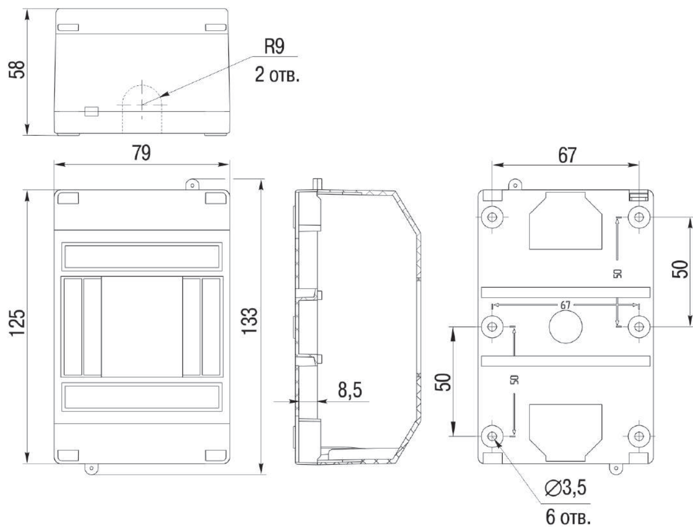
Рисунок 1 – Габаритные размеры корпусов КМПн 1/4
