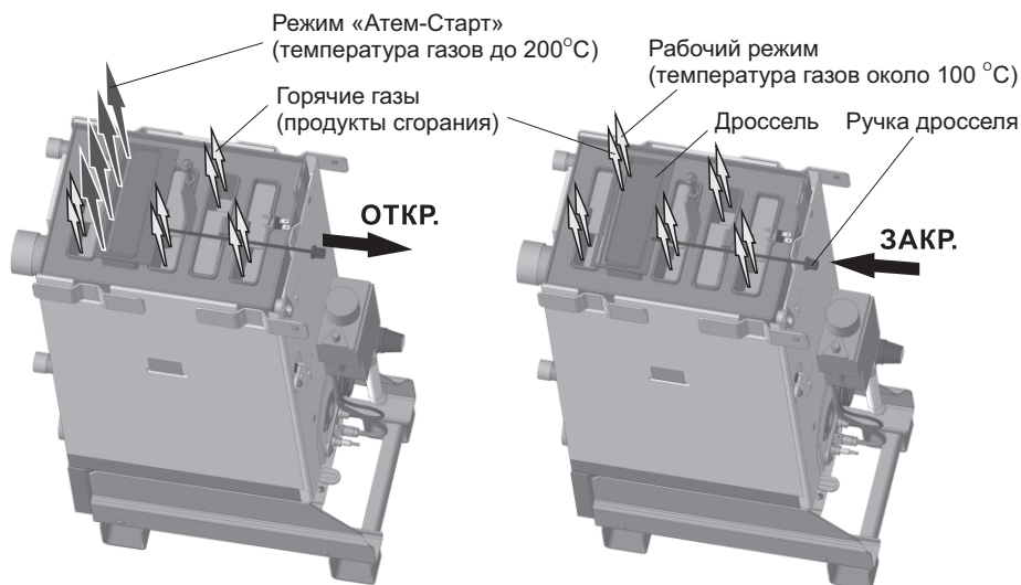
Рис. 12. система «Атем-старт»
