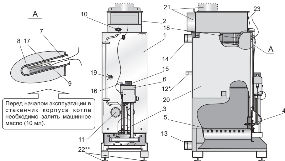
Рис. 1. Схема конструкции котла "Житомир-3" (декоративный кожух не показан)
