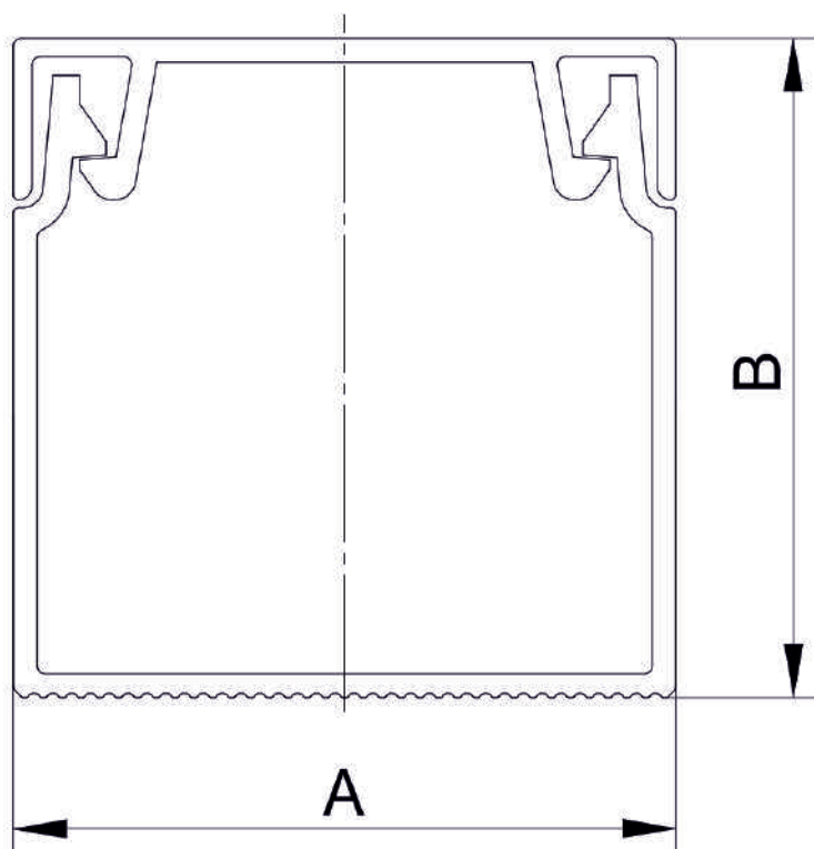
Габаритные размеры и площадь внутреннего поперечного сечения
