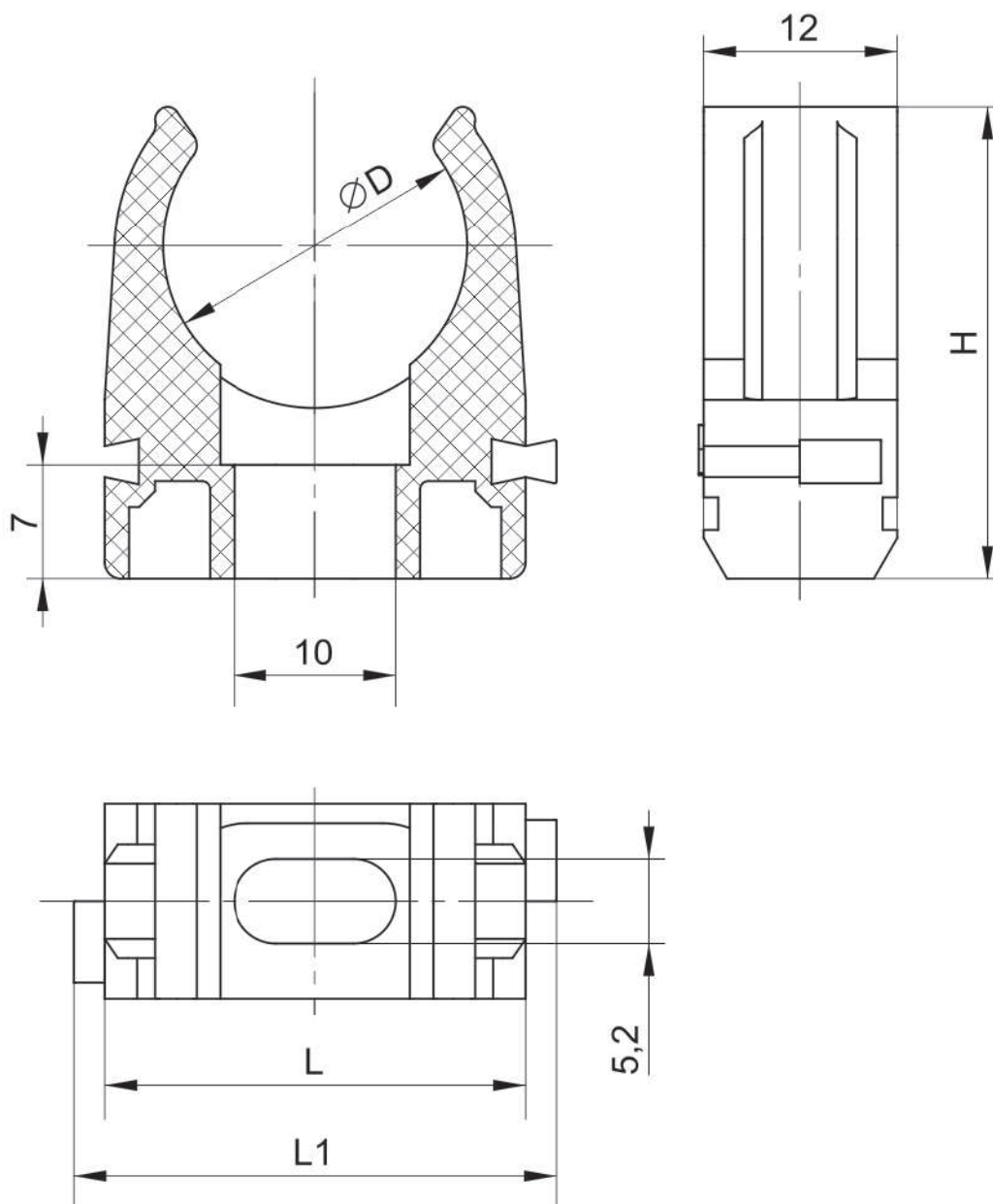
Рисунок 1 – Держатель с защёлкой
