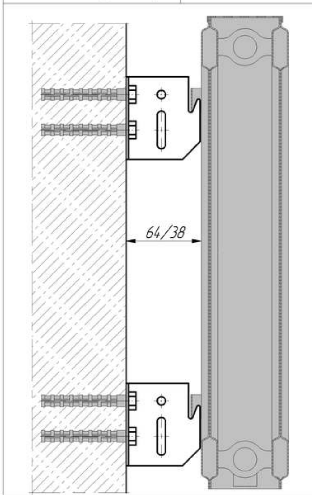
Схема монтажа радиатора
