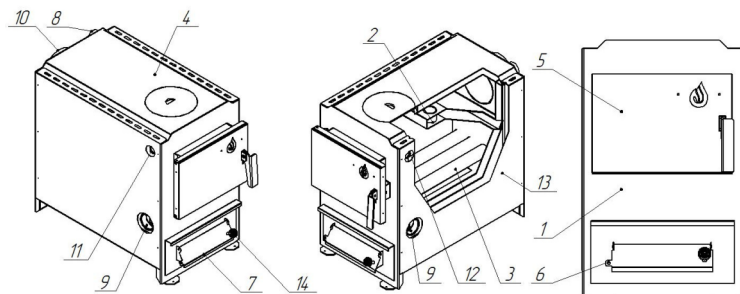
Рис 5. Устройство котла «РАТНИК» X180
