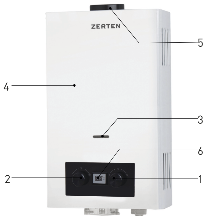
Рис. 1. Аппарат водонагревательный проточный газовый бытовой 1 – ручка водяного регулятора; 2 – ручка газового регулятора; 3 – окно смотровое; 4 – облицовка; 5 – патрубок дымоотвода; 6 – дисплей.
