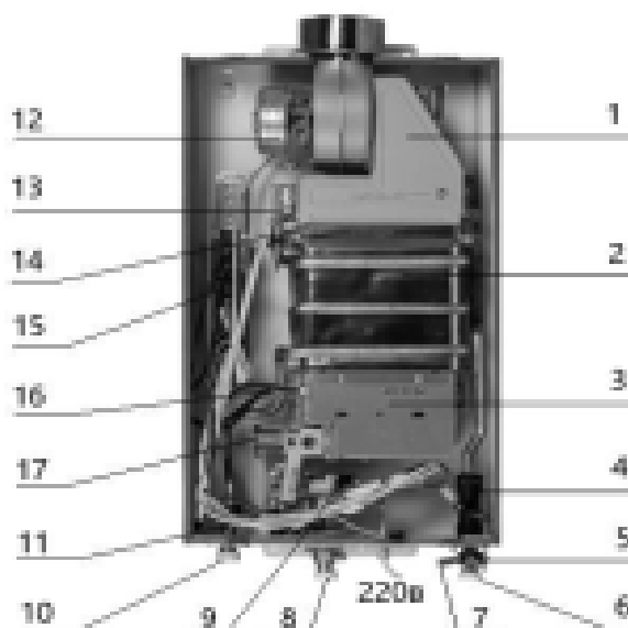
Рисунок 2. Внутренняя схема.
