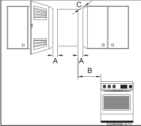
Рис. 12 Минимальные расстояния
