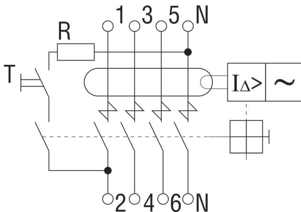
Схема электрическая принципиальная четыреполюсных выключателей
