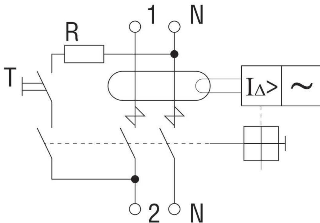
Схема электрическая принципиальная двухполюсных выключателей
