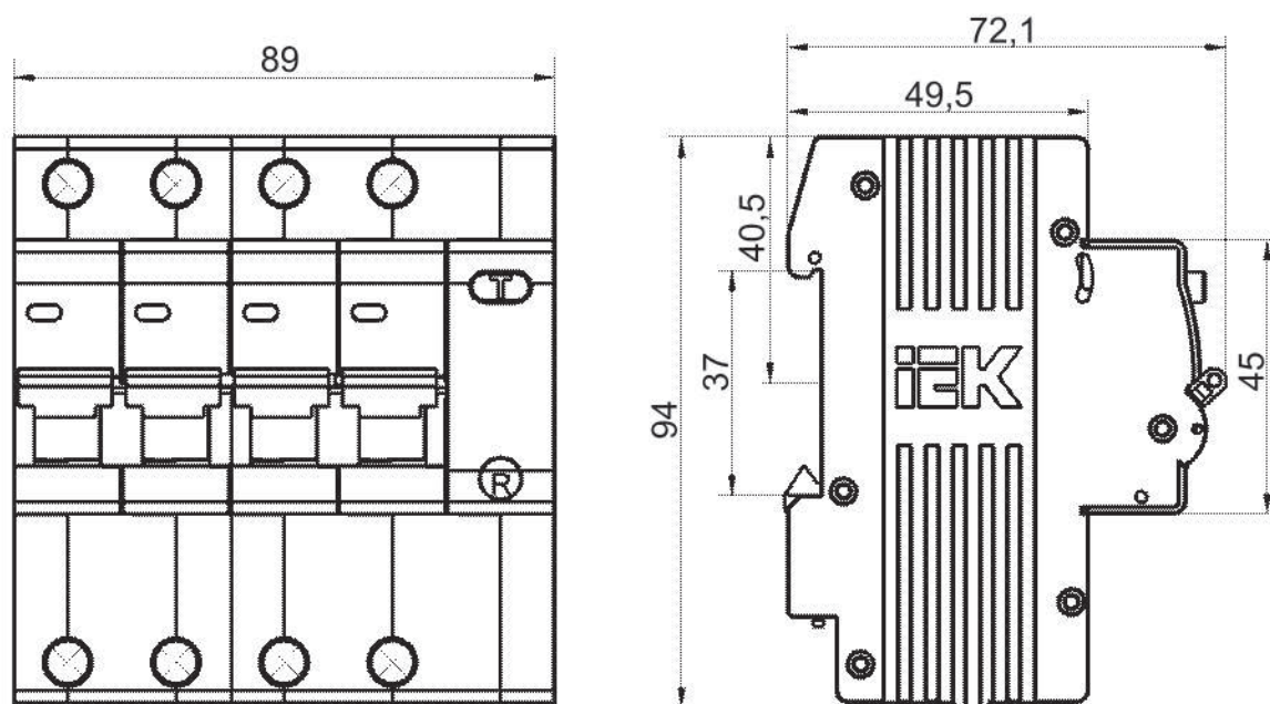
Рисунок 2. Габаритные размеры АД14
