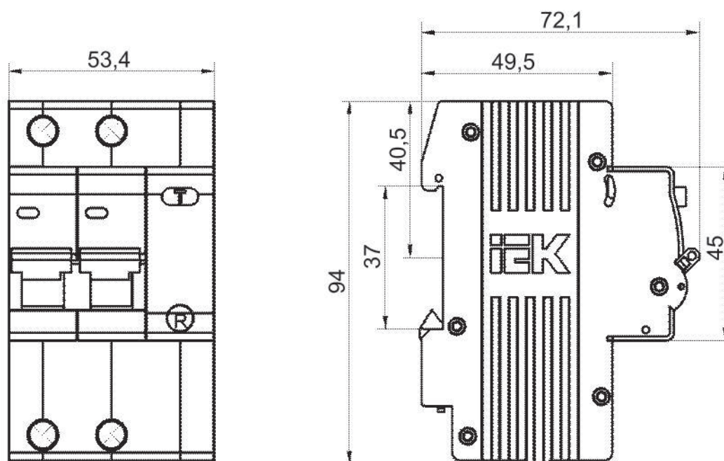
Рисунок 1. Габаритные размеры АД12
