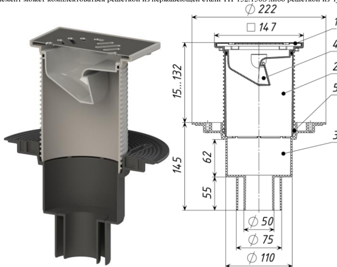
Рис. 1 ТП-310N Трап с незамерзающим запахозапирающим устройством
